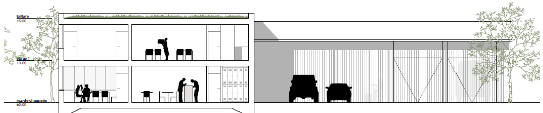
coupe A échelle 1: 200
