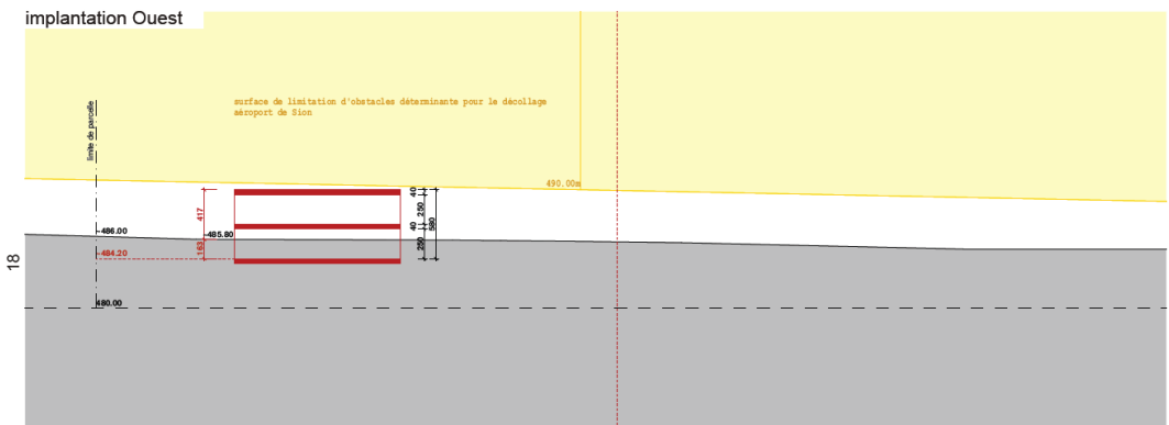
coupe projet sur 2 niveaux, à l'Ouest, excavé échelle 1: 500
